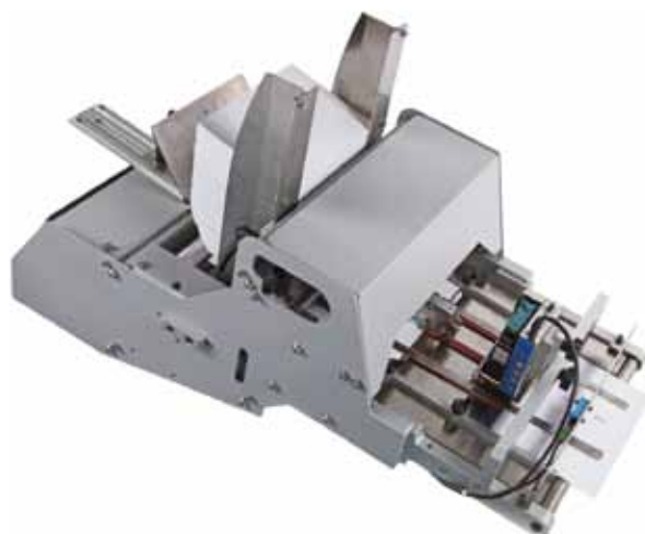
FEEDER - podavač vkladů, lístků
