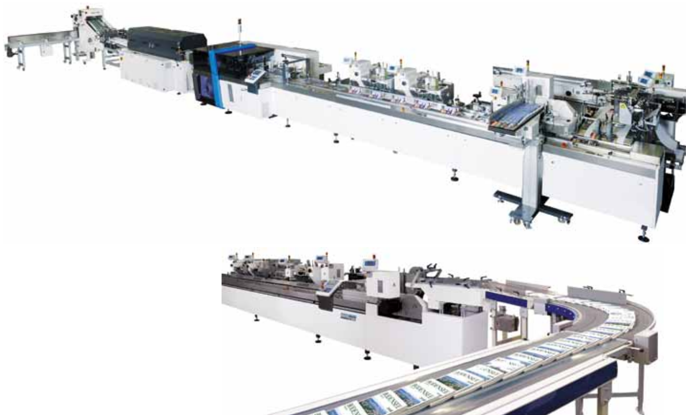
Automatická balicí linka vč. dávkovačů, značení, tunelu a stohovače na výstupu
